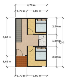
Lantai 2
